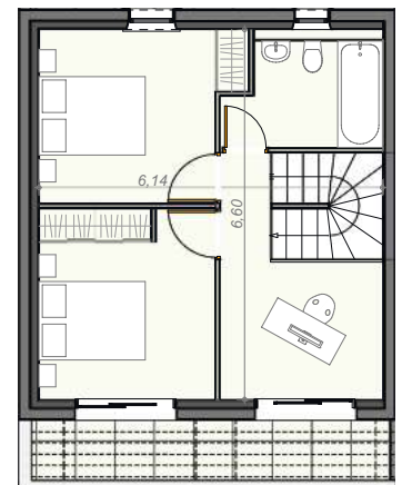
Plan Etage 3
