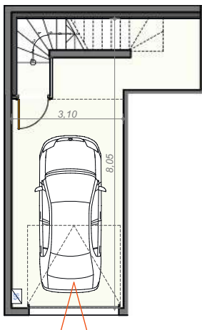
Plan Rez de chaussée
