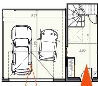
Plan Rez de chaussée
