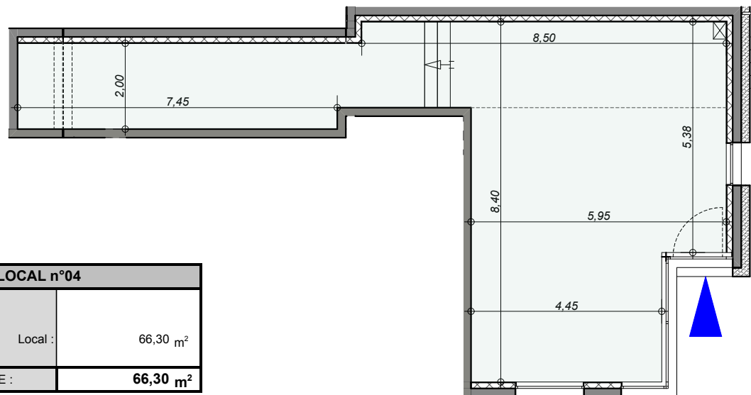
PLAN DU LOCAL en Rez de Chaussée
